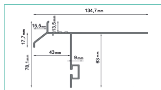
K40 DRIP EDGE
