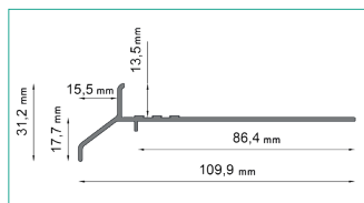
K30 DRIP EDGE
