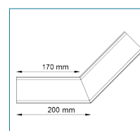
RK65 135 INTERNAL GUTTER ANGLE
