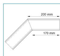
RK65 135 EXTERNAL GUTTER ANGLE
