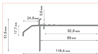
K20R DRIP EDGE
