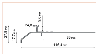
K20 DRIP EDGE
