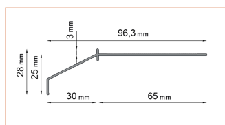
K10 DRIP EDGE
