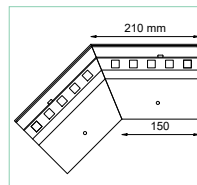
NAROŻNIK ZEWNĘTRZNY W20R 135
