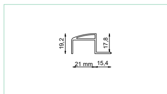
PROFIL ZAMYKAJĄCY W20Z
