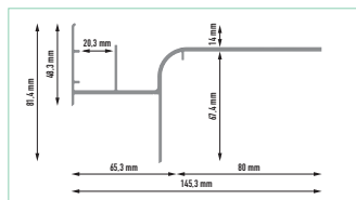
PROFIL OKAPOWY W20R
