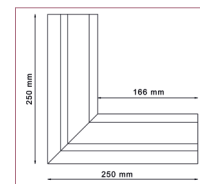
NAROŻNIK WEWNĘTRZNY C2 90 PIONOWY
